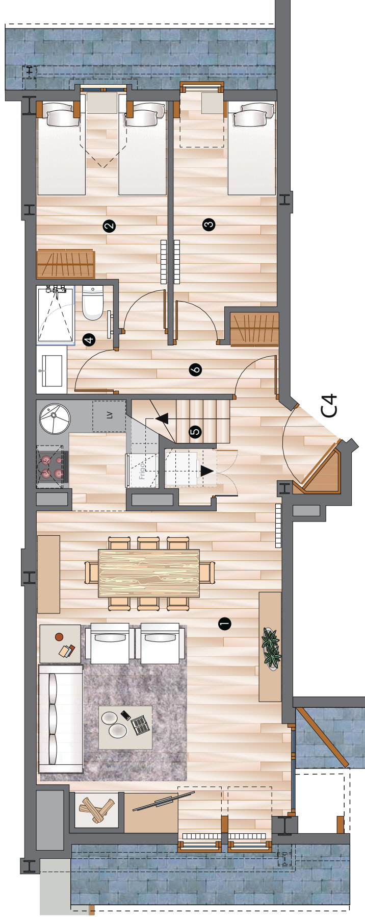
Planta bajocubierta / attic floor
