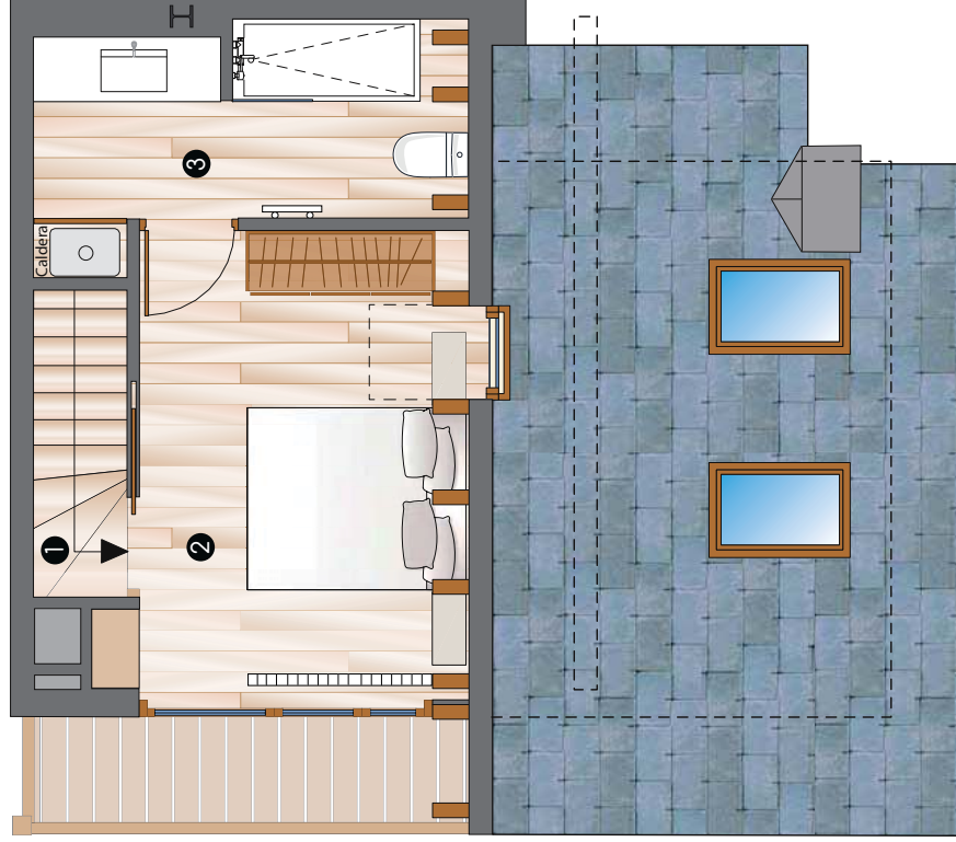
Planta bajocubierta / attic floor
